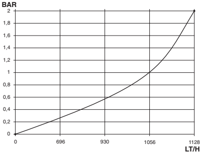
DIAGRAMMA PERDITE DI CARICO PRESSURE LOSS CHARACTERISTICS
